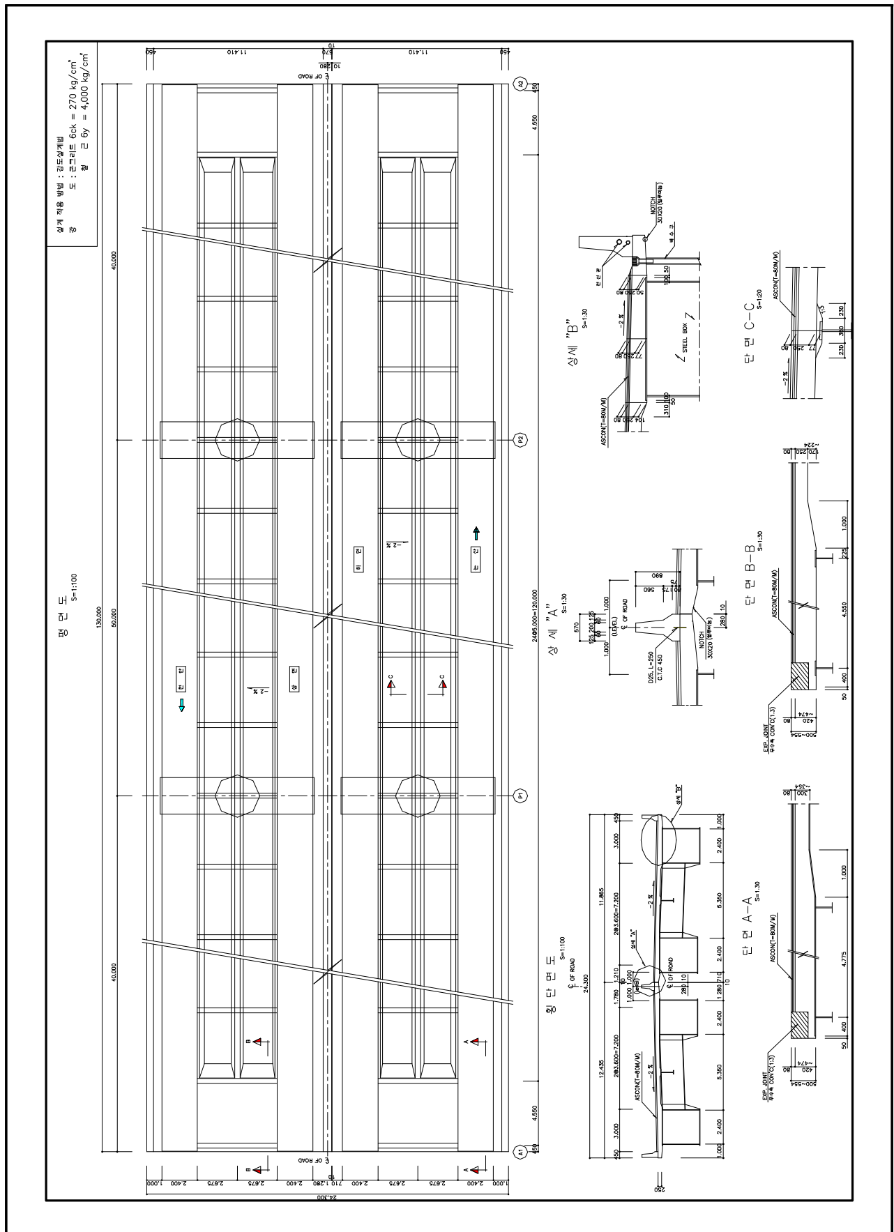
【그림 1.4】 슬래브 일반도
